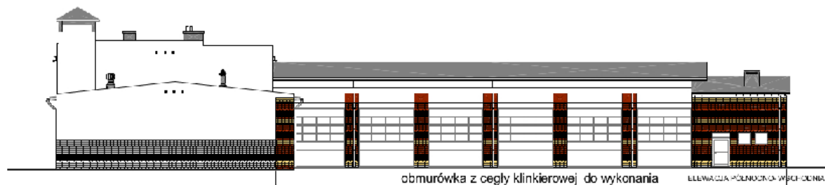
ELEWACJA PÓŁNOCNO-WSCHODNIA
