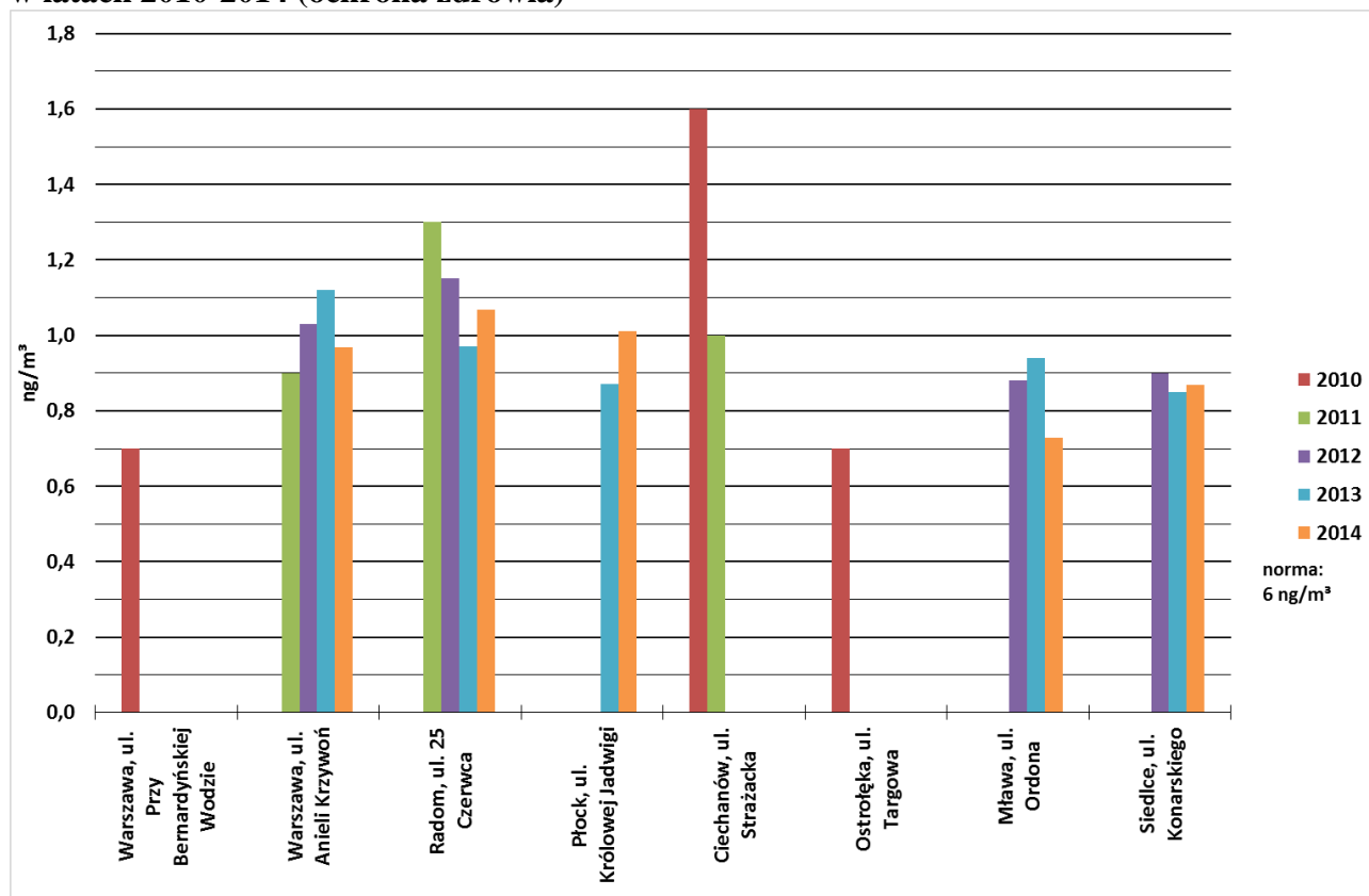
WYKRES Z4-12. Wartości stężeń średniorocznych arsenu w województwie mazowieckim w latach 2010-2014 (ochrona zdrowia)
