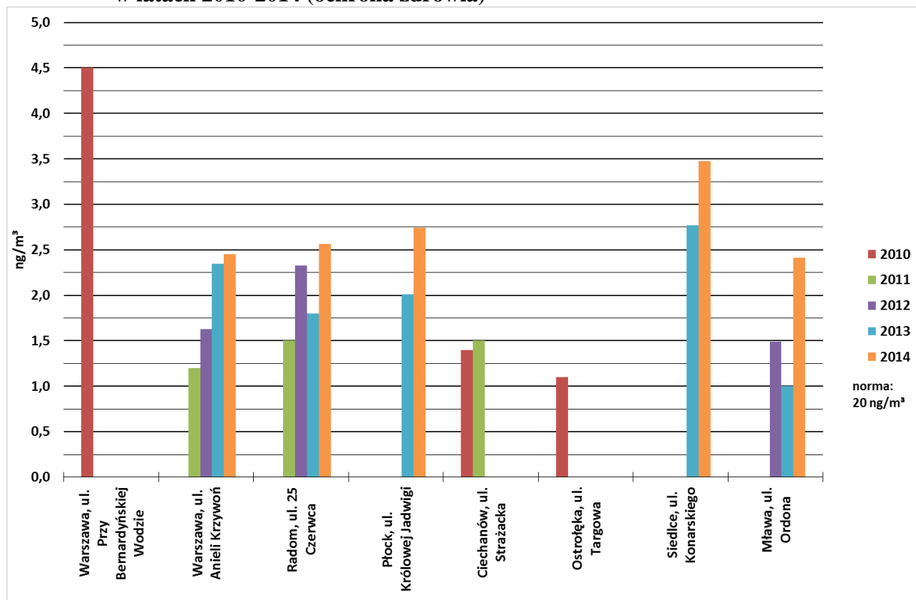
WYKRES Z4-14. Wartości stężeń średniorocznych niklu w województwie mazowieckim w latach 2010-2014 (ochrona zdrowia)
