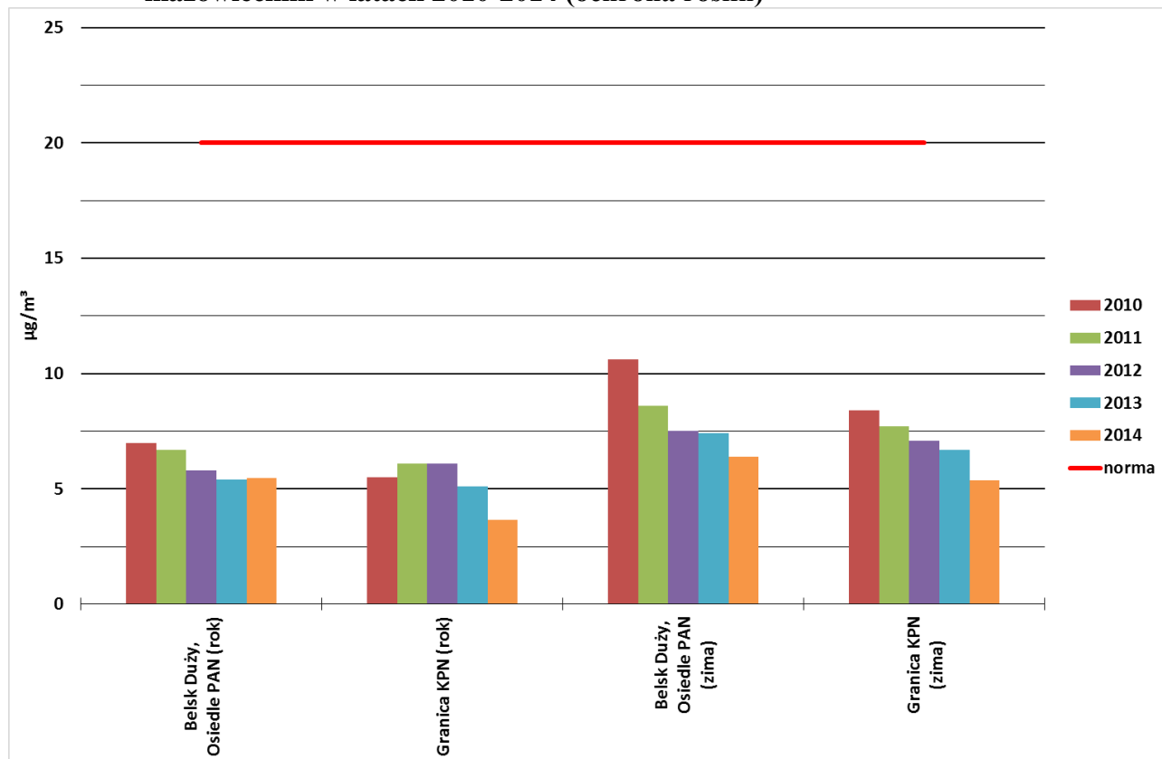
WYKRES Z4-18. Wartości stężeń średniorocznych i średnio zimowych SO 2 w województwie mazowieckim w latach 2010-2014 (ochrona roślin)
