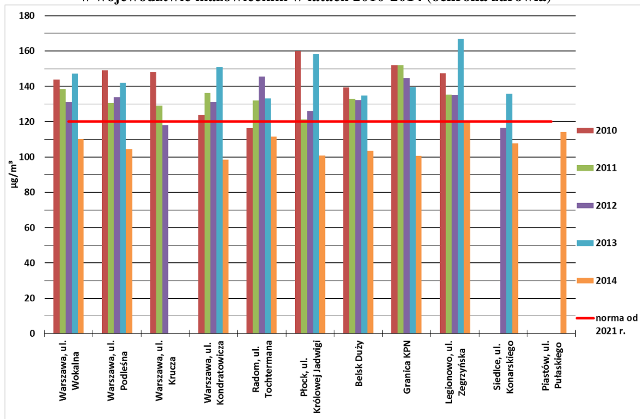
WYKRES Z4-17. Wartości stężeń 26-tego maksimum ze stężeń 8-godzinnych O 3 w województwie mazowieckim w latach 2010-2014 (ochrona zdrowia)
