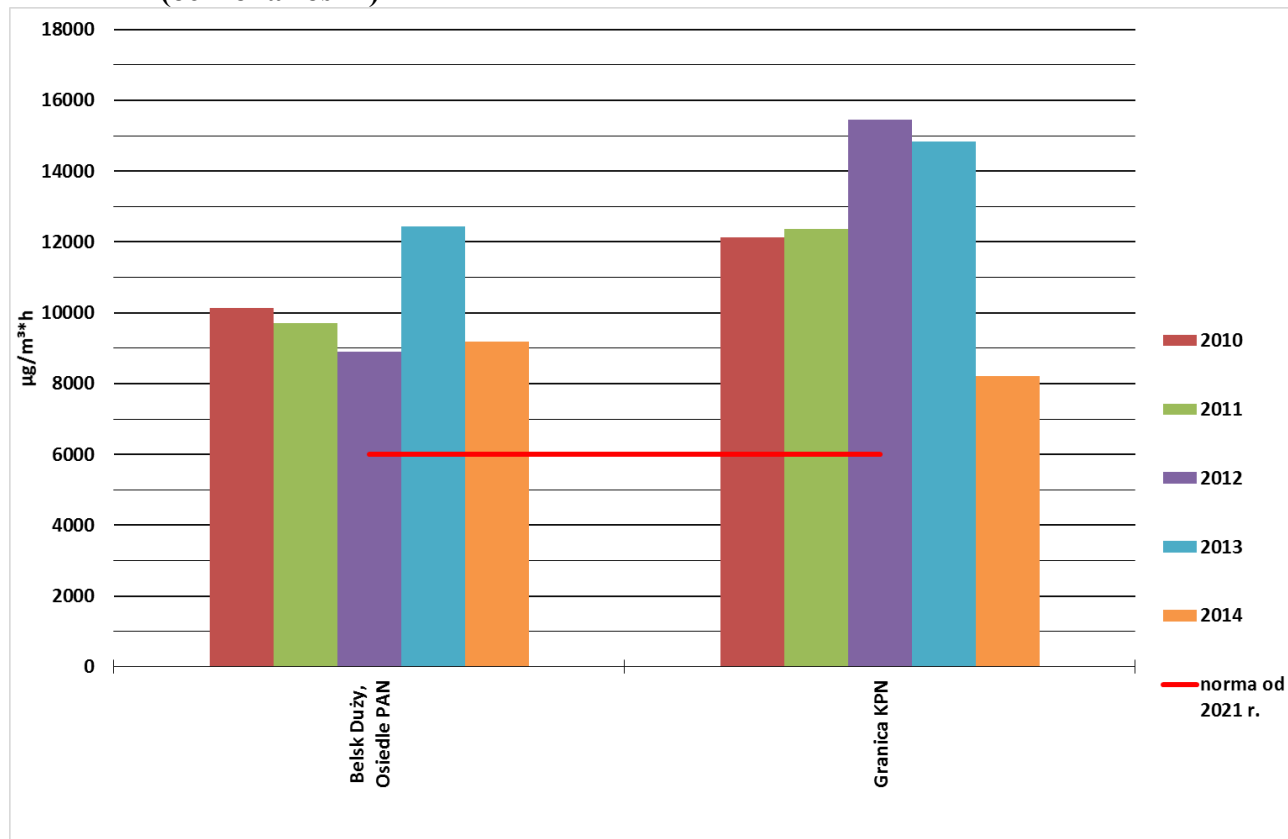
WYKRES Z4-20. Wartości stężeń AOT40 w województwie mazowieckim w latach 2010-2014 (ochrona roślin)
