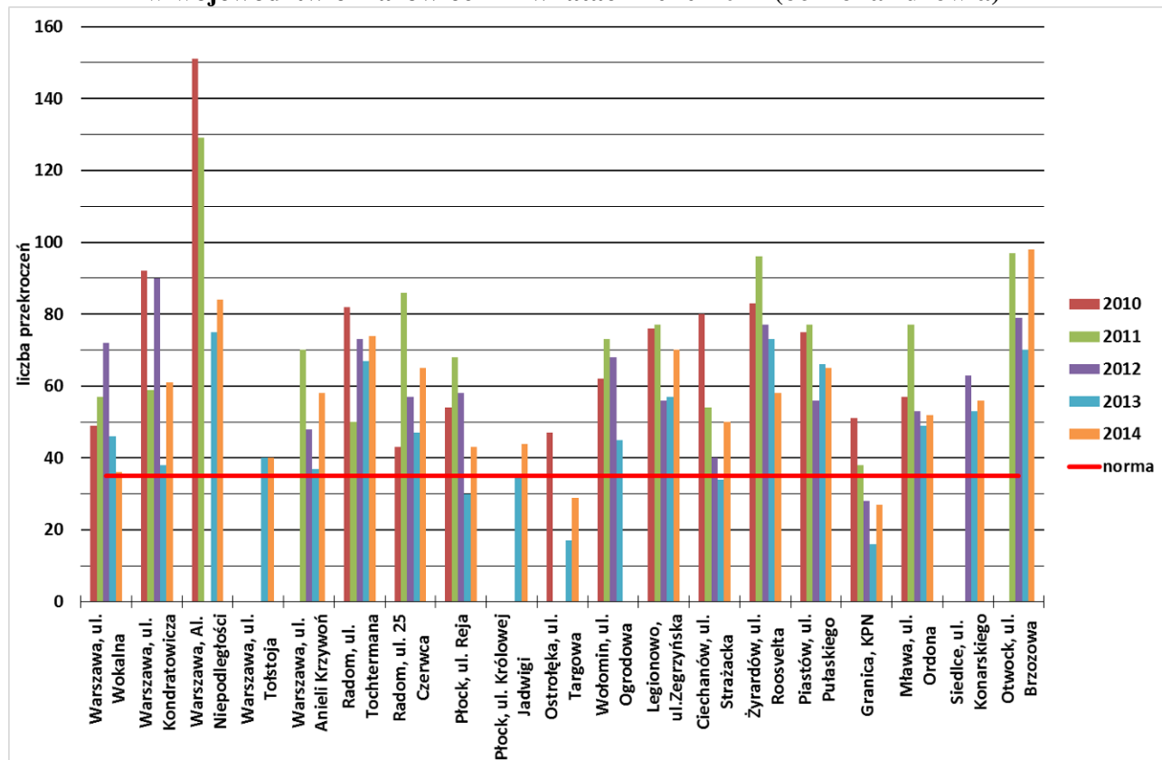
WYKRES Z4-9. Liczba dni z przekroczeniem normy dobowej pyłu zawieszonego PM10 w województwie mazowieckim w latach 2010-2014 (ochrona zdrowia)
