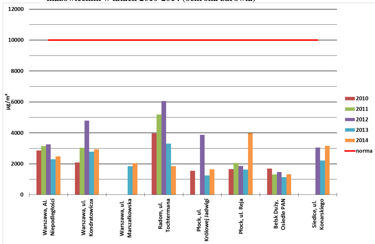
WYKRES Z4-6. Wartość maksymalnego stężenia 8-godzinnego CO w województwie mazowieckim w latach 2010-2014 (ochrona zdrowia)
