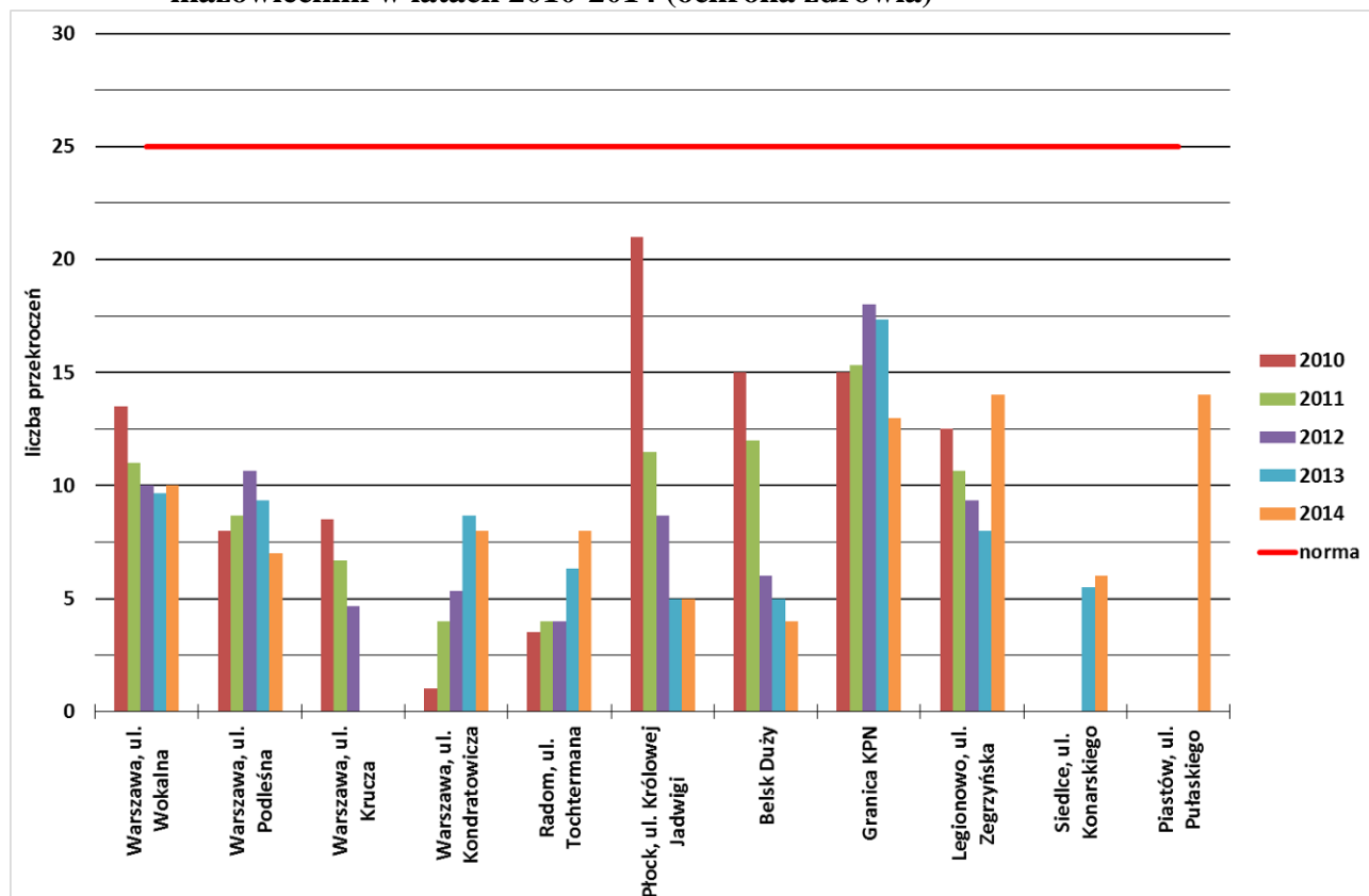
WYKRES Z4-16. Liczba dni z przekroczeniem normy 8-godzinnej O 3 w województwie mazowieckim w latach 2010-2014 (ochrona zdrowia)
