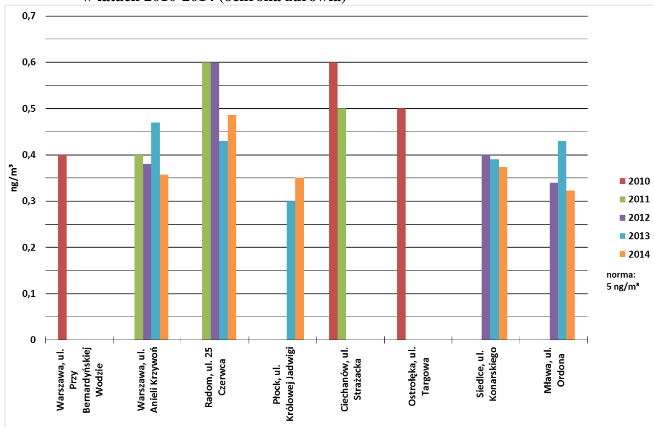
WYKRES Z4-13. Wartości stężeń średniorocznych kadmu w województwie mazowieckim w latach 2010-2014 (ochrona zdrowia)
