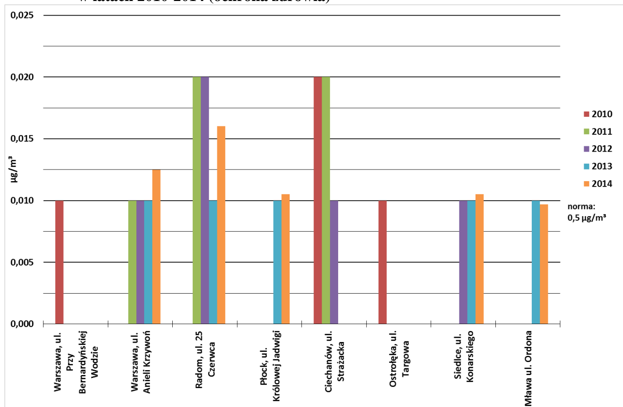
WYKRES Z4-11. Wartości stężeń średniorocznych ołowiu w województwie mazowieckim w latach 2010-2014 (ochrona zdrowia)
