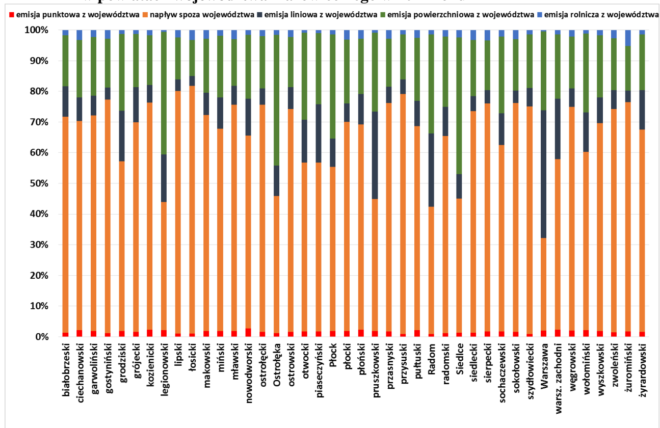
WYKRES Z4-22. Udział poszczególnych źródeł emisji w stężeniu średniorocznym PM10 w powiatach województwa mazowieckiego w 2014 roku
