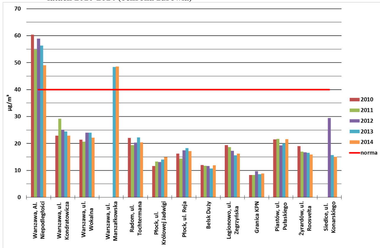
WYKRES Z4-4. Wartości stężeń średniorocznych NO 2 w województwie mazowieckim w latach 2010-2014 (ochrona zdrowia)
