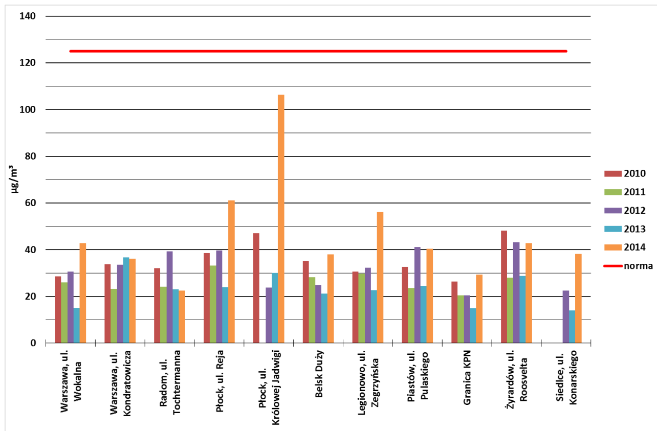
WYKRES Z4-2. Wartości stężeń 4-tego maksimum ze stężeń 24-godzinnych SO 2 w województwie mazowieckim w latach 2010-2014 (ochrona zdrowia)
