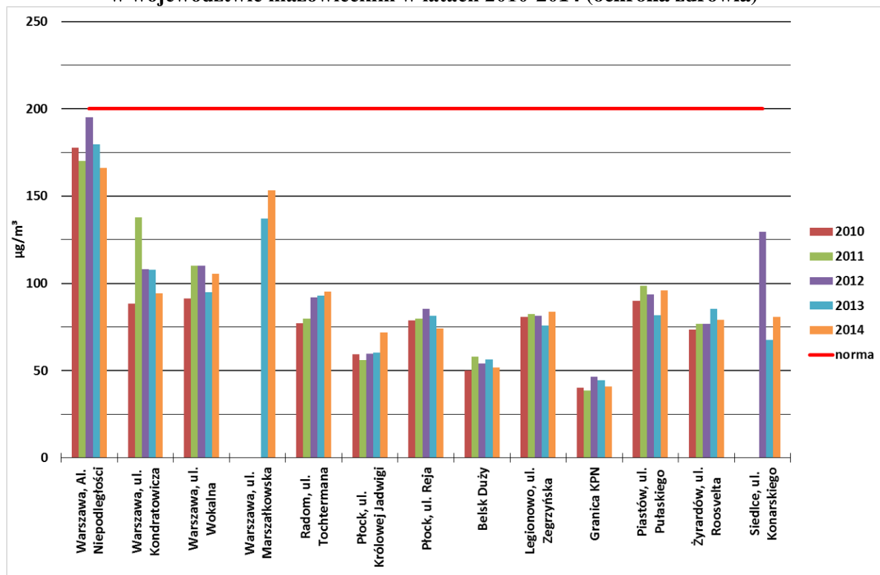
WYKRES Z4-5. Wartości stężeń 19-tego maksimum ze stężeń 1-godzinnych NO 2 w województwie mazowieckim w latach 2010-2014 (ochrona zdrowia)
