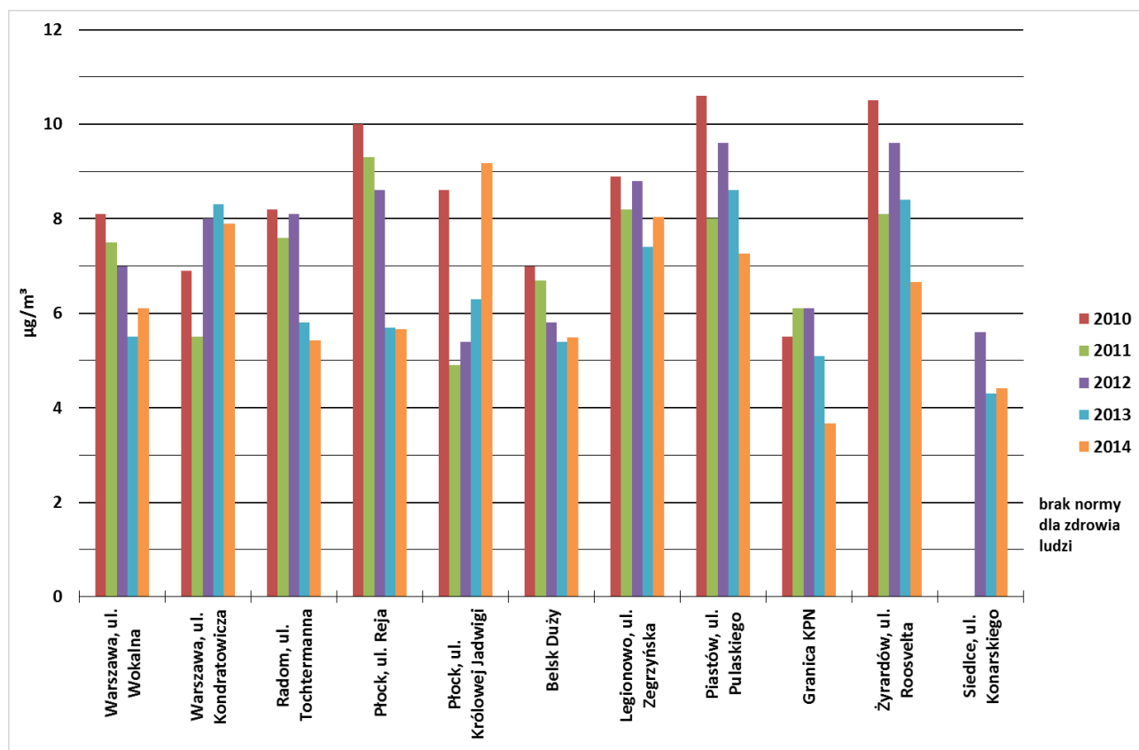
WYKRES Z4-4. Wartości stężeń średniorocznych NO 2 w województwie mazowieckim w latach 2010-2014 (ochrona zdrowia)
