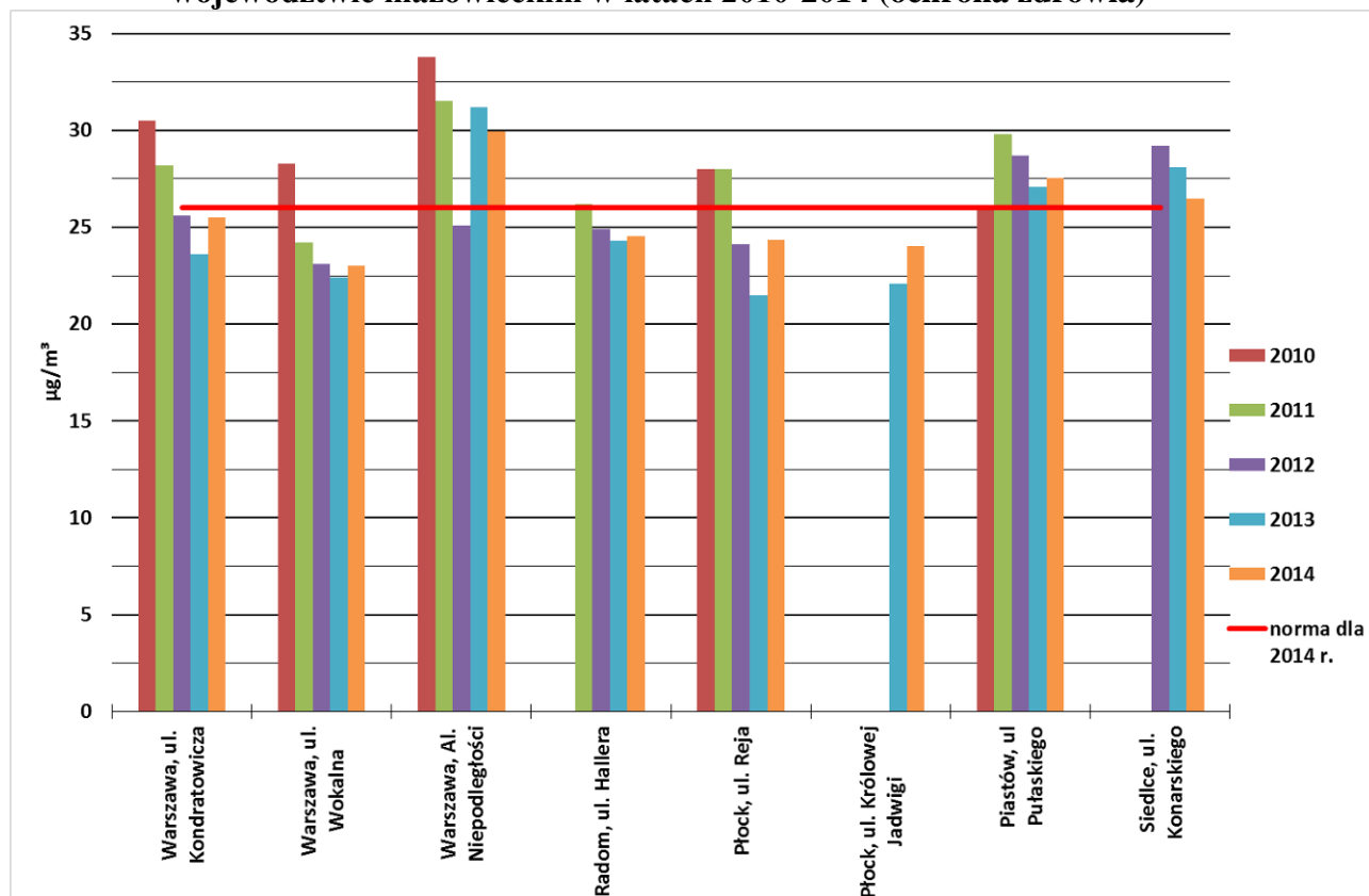
WYKRES Z4-10. Wartości stężeń średniorocznych pyłu zawieszonego PM2,5 w województwie mazowieckim w latach 2010-2014 (ochrona zdrowia)
