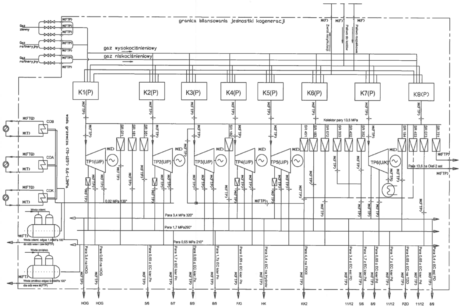
Rysunek 5-1 Schemat technologiczny
